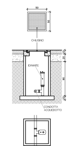
PARTICOLARE POZZETTO CON IDRANTE
