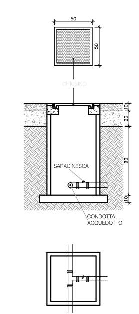
PARTICOLARE POZZETTO
